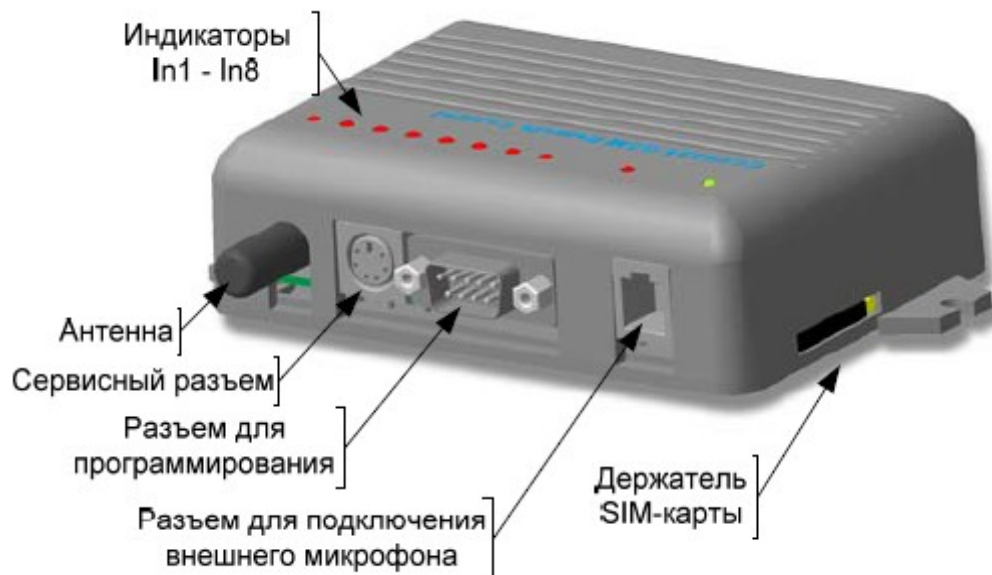
Рисунок 1. CCU6225 – основные элементы, сервисный разъем может отсутствовать
